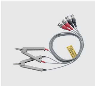
4端子探棒9140-10 4端子探棒9140 測試線零件用 可測量端子直徑: 0.3~5 mm 連接線長: 1 m
