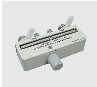
測試治具9262 測試線零件用 可測量端子直徑: 0.3~2 mm 測試線的Pitch: 5 mm以上 測量主機直連類型
