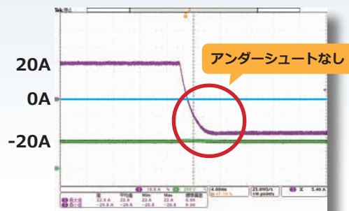
DC SEAM モードの動作例
